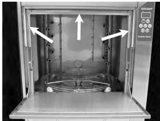
obraz 44 Ramka drzwi do wyczyszczenia.
