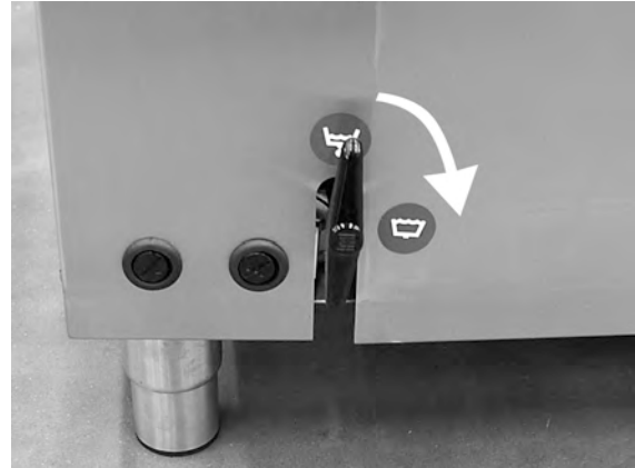
Bild 3 Tömningsventil
