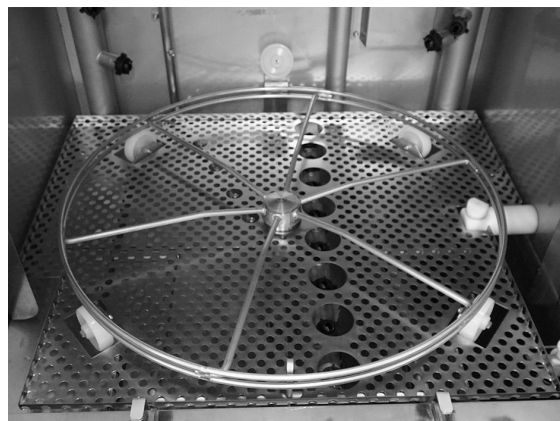
Abbildung 4 Korbrad
