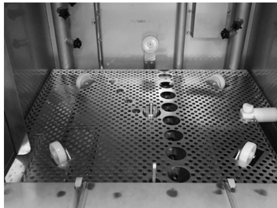
Abbildung 3 Tankgitter
