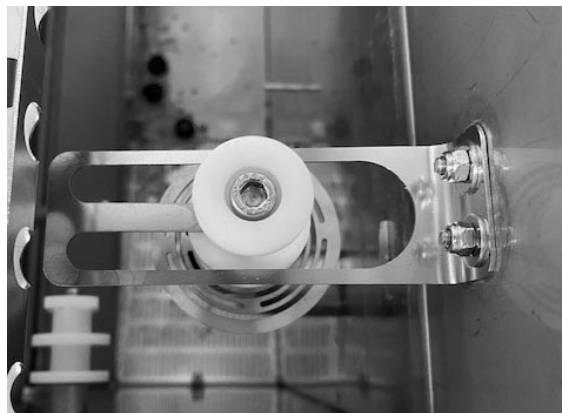
Abbildung 40 Überlaufarmatur
