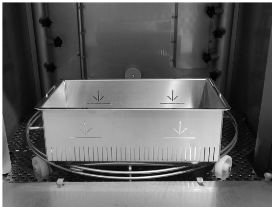
Obrázek 32 Sběrač granulí uvnitř myčky
