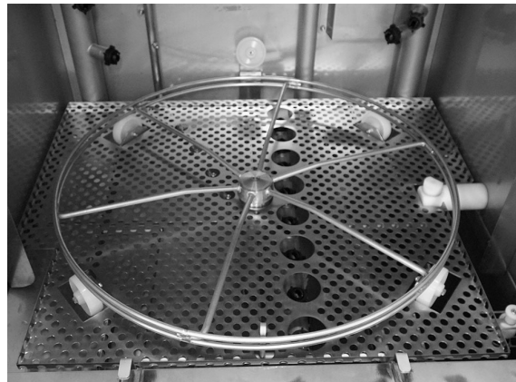
Kuva 4 Koripyörä
