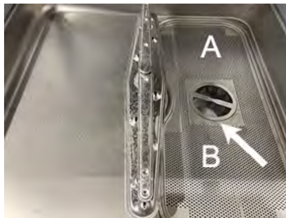
Imagine 10 Scoaterea plasei și filtrului de rezervor
